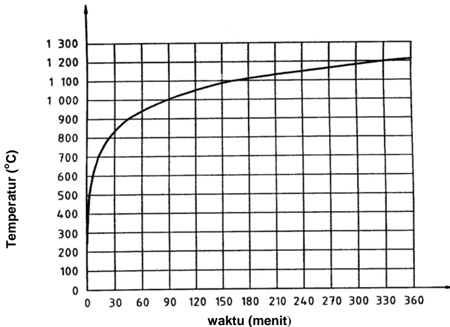
Gambar 4 Kurva waktu-temperatur standar
