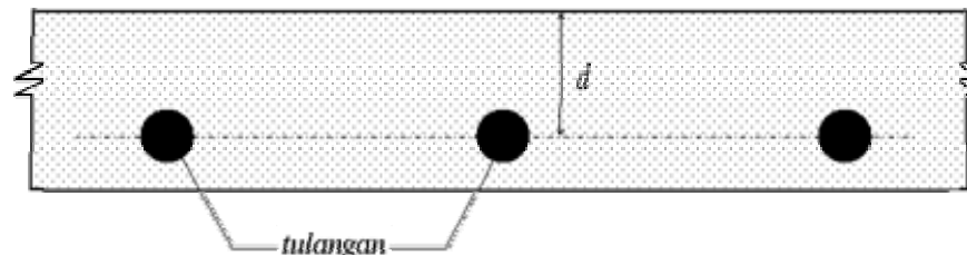
Gambar B.3 Ilustrasi jarak d pada beton
